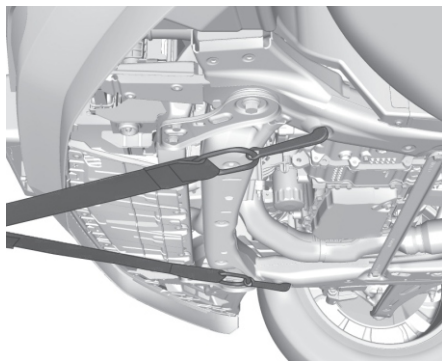
Передние точки крепления
